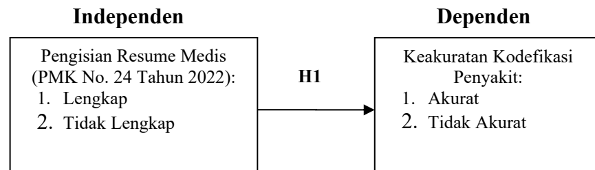
Gambar 3.1 Kerangka Konseptual
