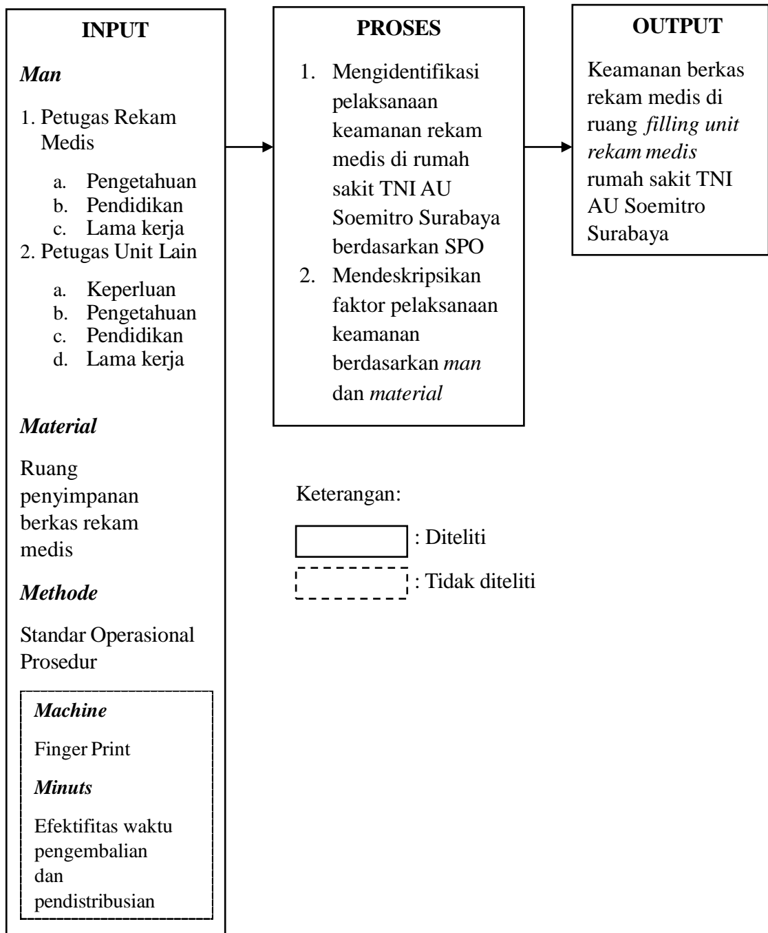
Gambar 3.1 Kerangka Konseptual
