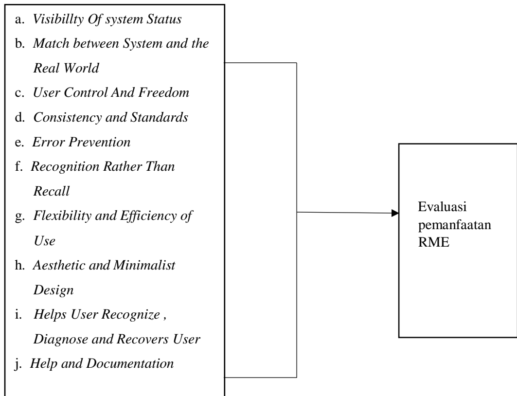
Gambar 3.1 Kerangka konseptual
