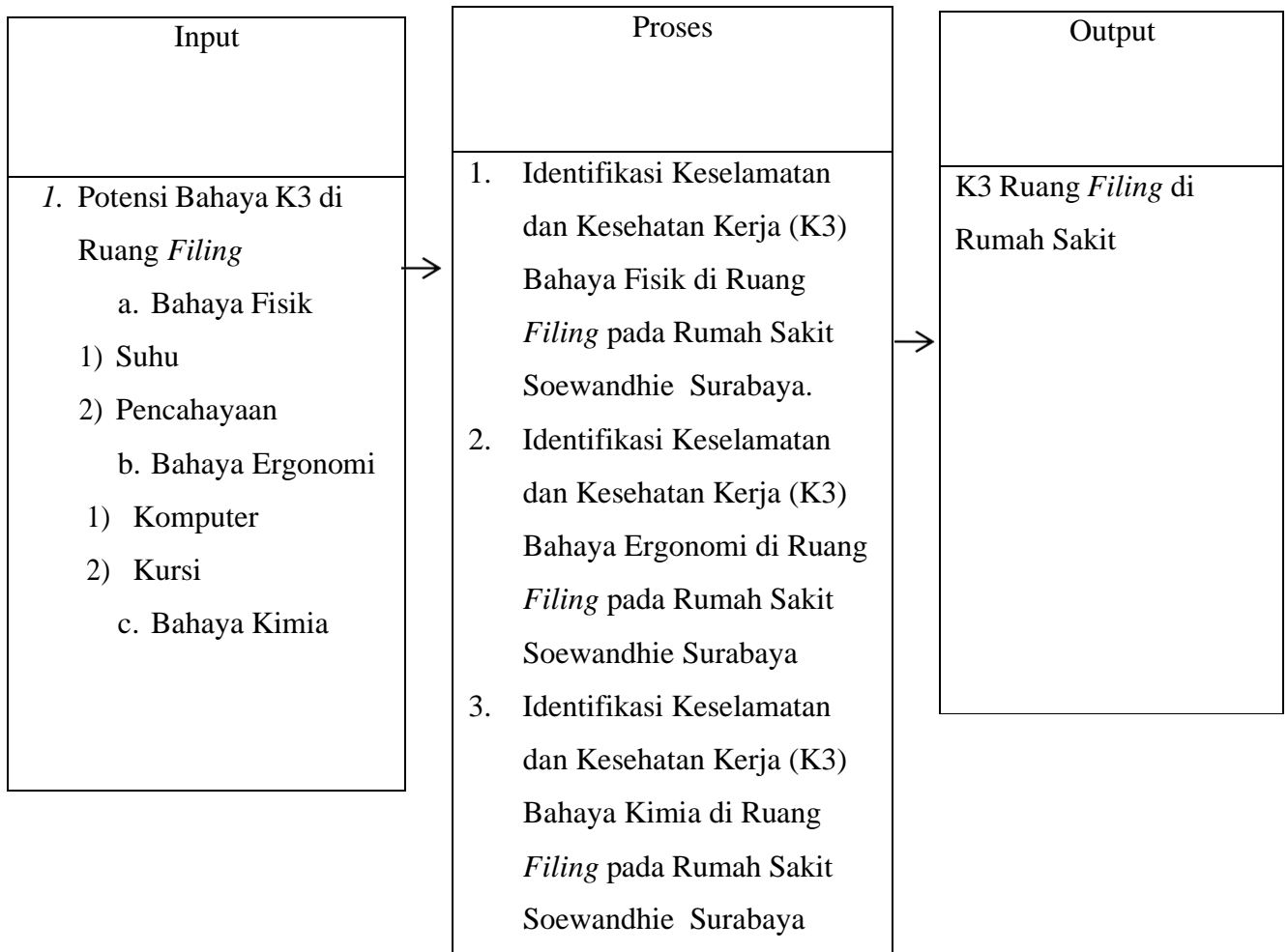
Gambar 3.1 Kerangka Konseptual
