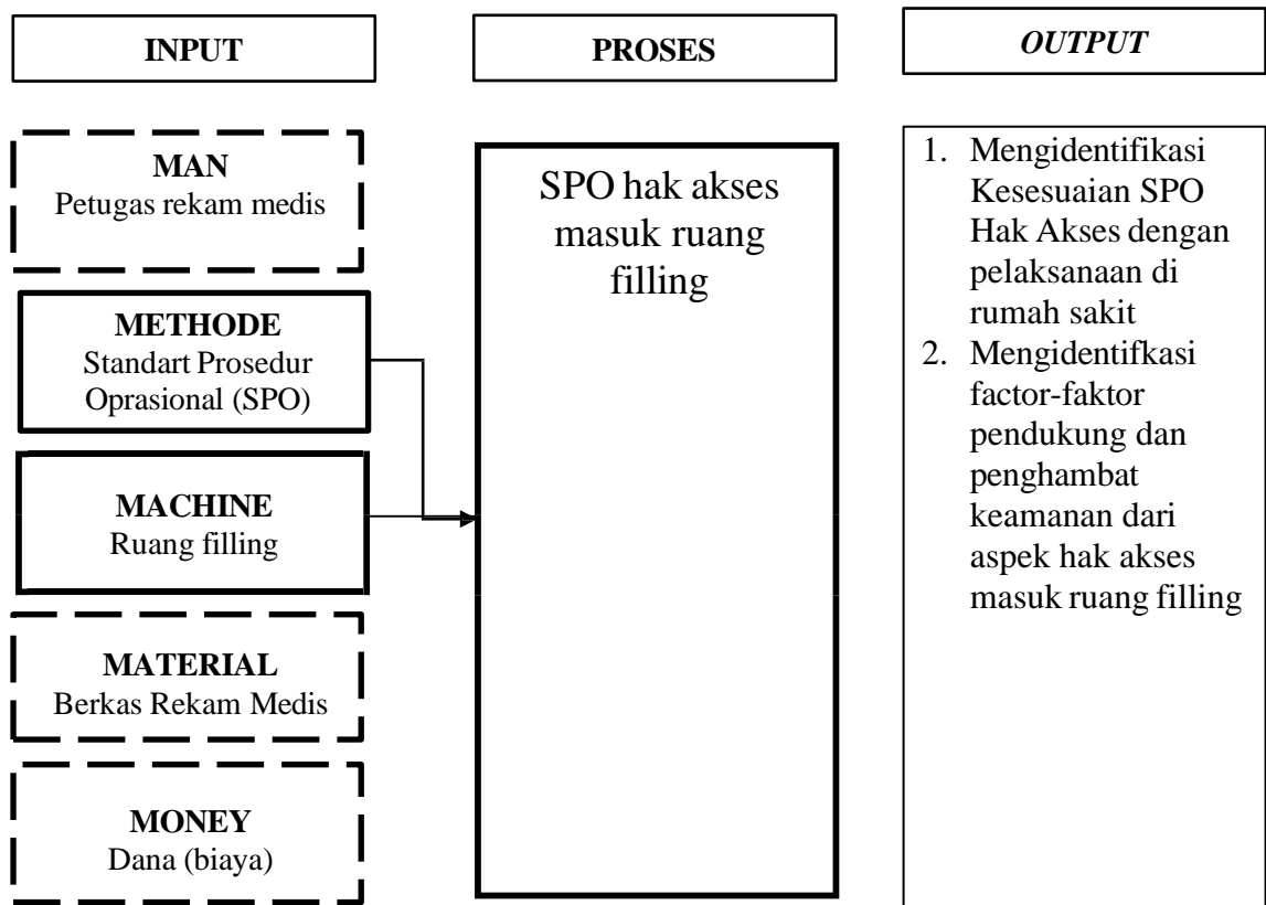
Gambar 3.1 Kerangka Konseptual
