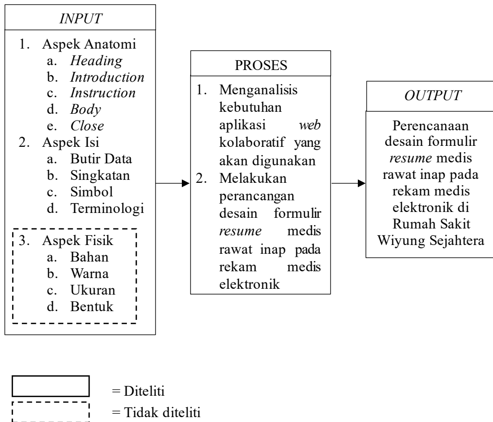
Gambar 3.1 Kerangka Konseptual
