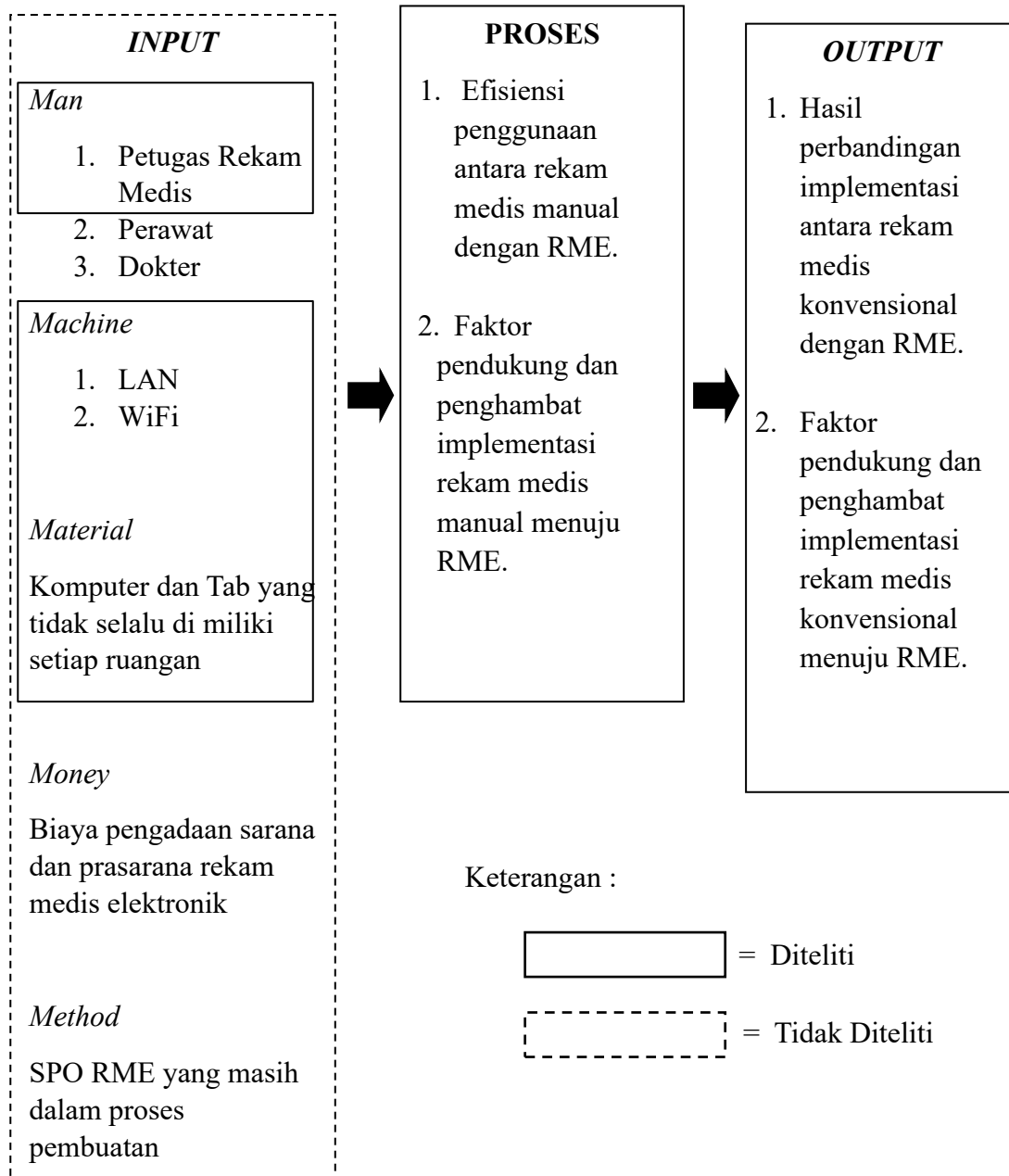
Gambar 3.1 Kerangka Konseptual
