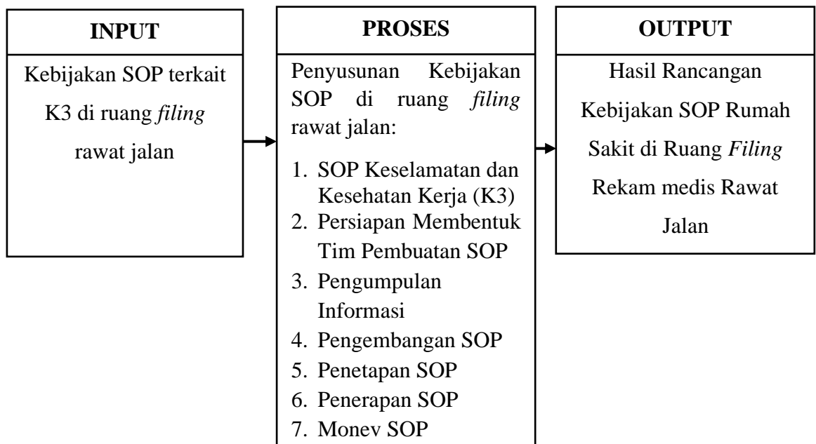
Gambar 3.1 Kerangka Konseptual
