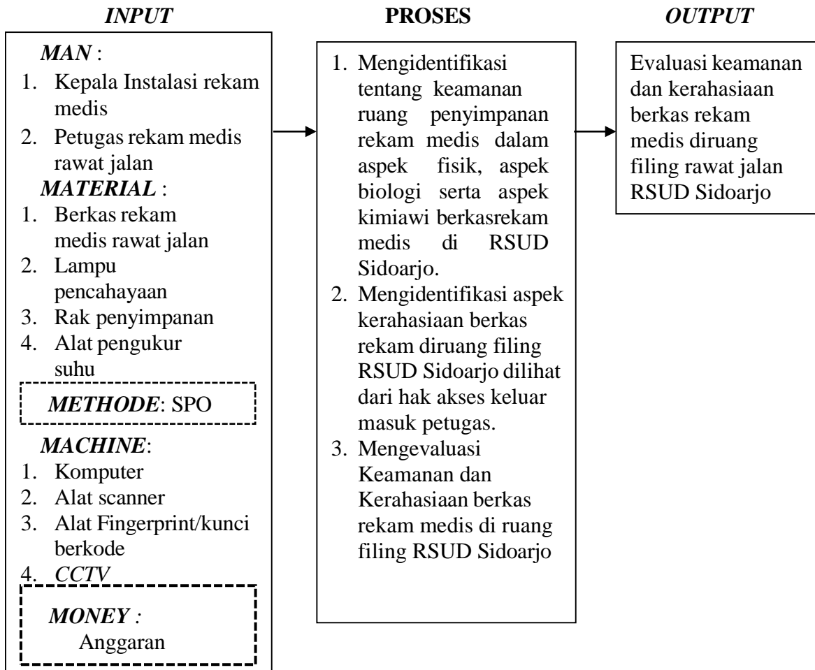
Gambar 3.1 Kerangka Konseptual
