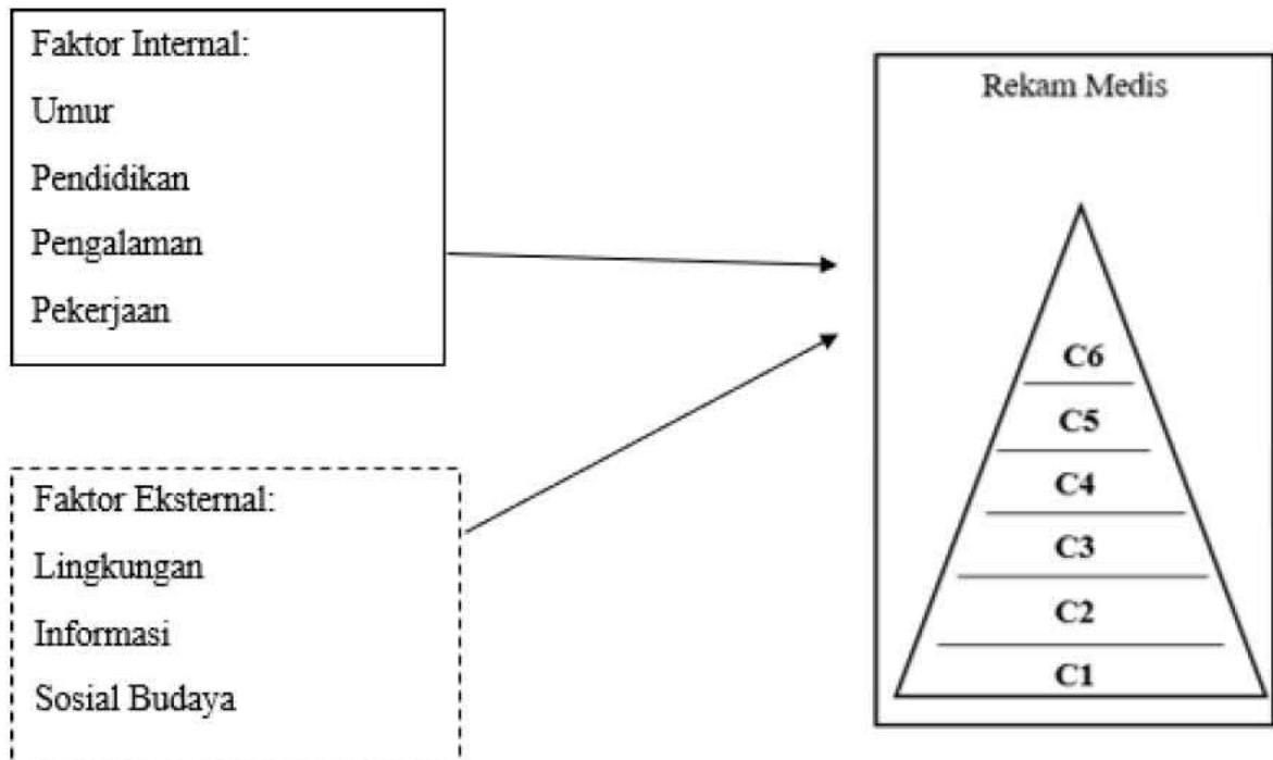
Gambar 3.1 Kerangka Konseptual
