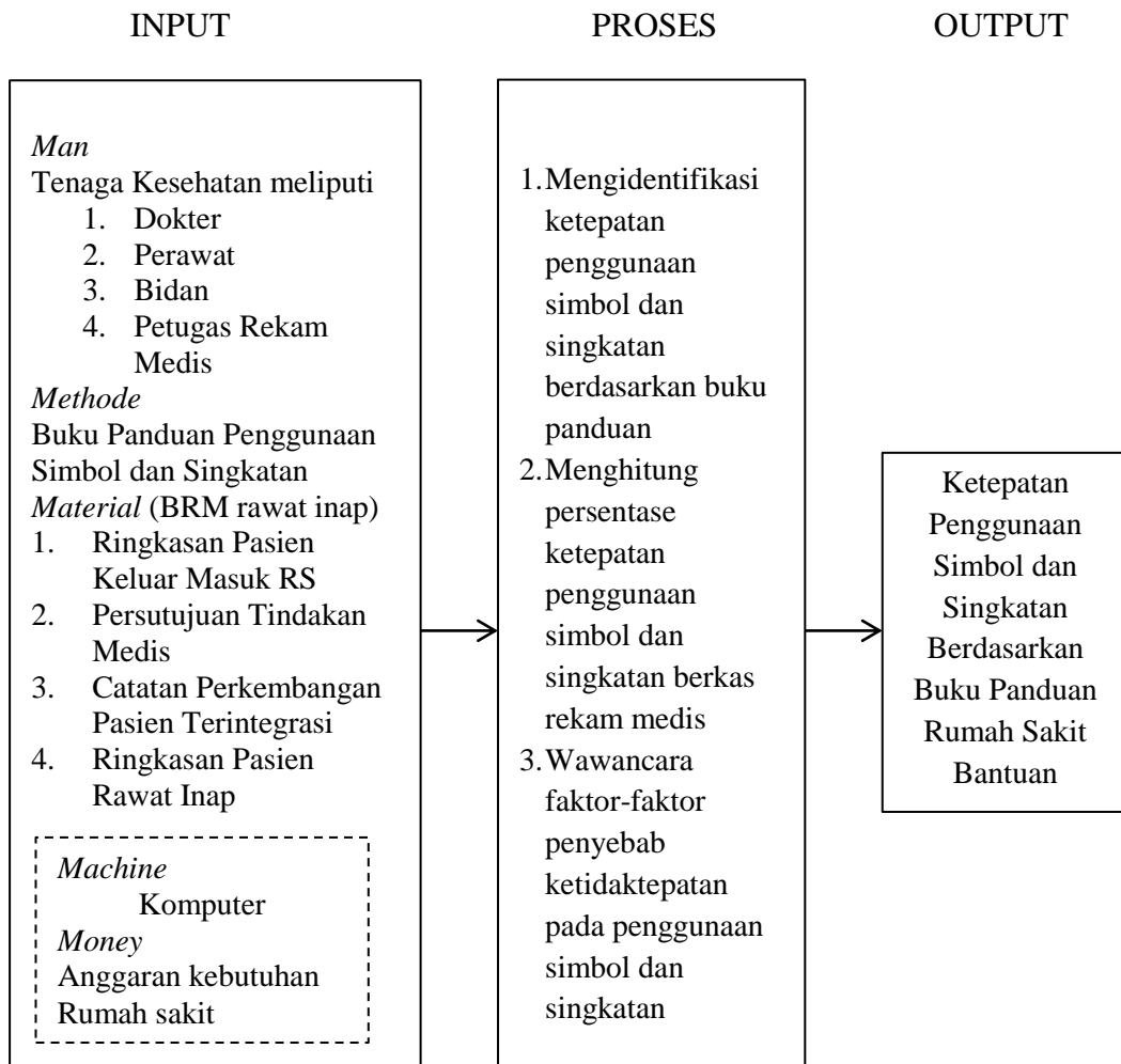
Gambar 3. 1 Kerangka Konseptual
