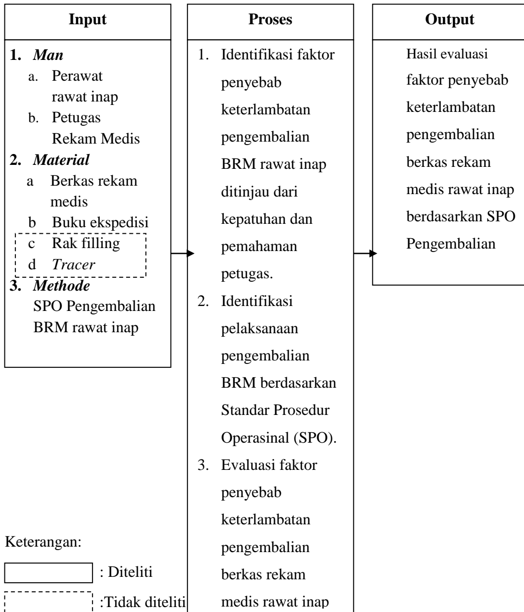
Gambar 3. 1 Kerangka Konseptual
