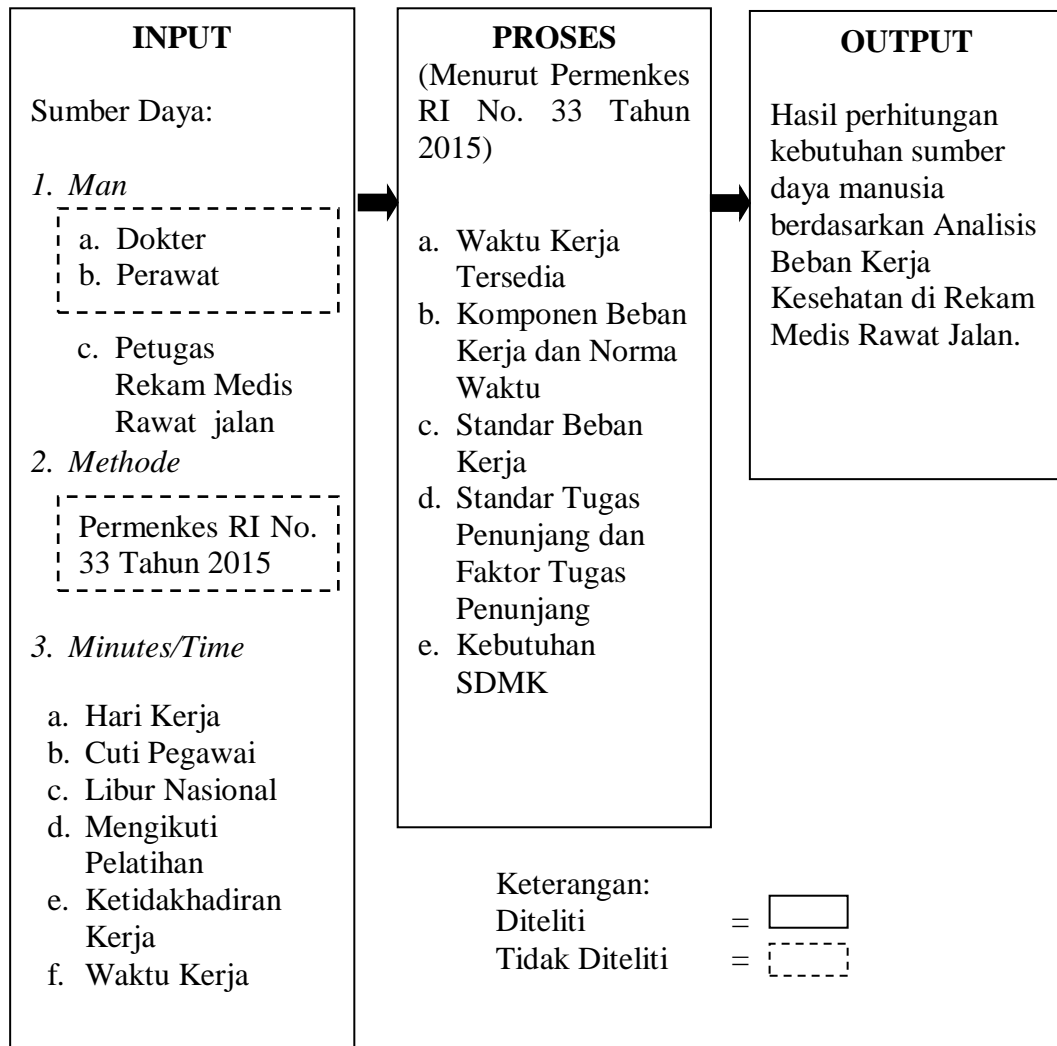
Gambar 3.1 Kerangka Konseptual
