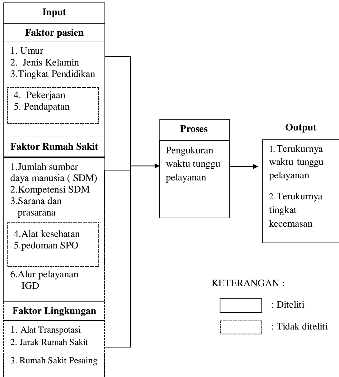
Gambar 3.1 Kerangka Konseptual
