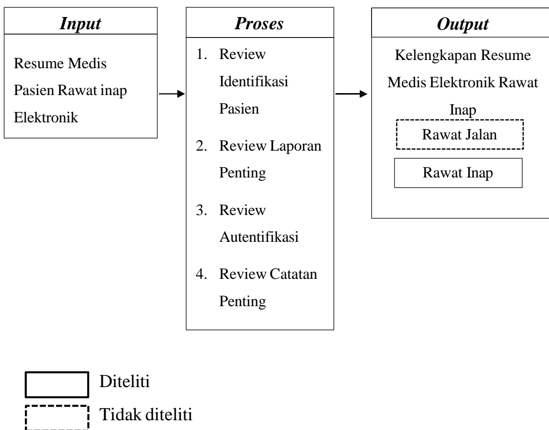
Gambar 3.1 Kerangka Konseptual
