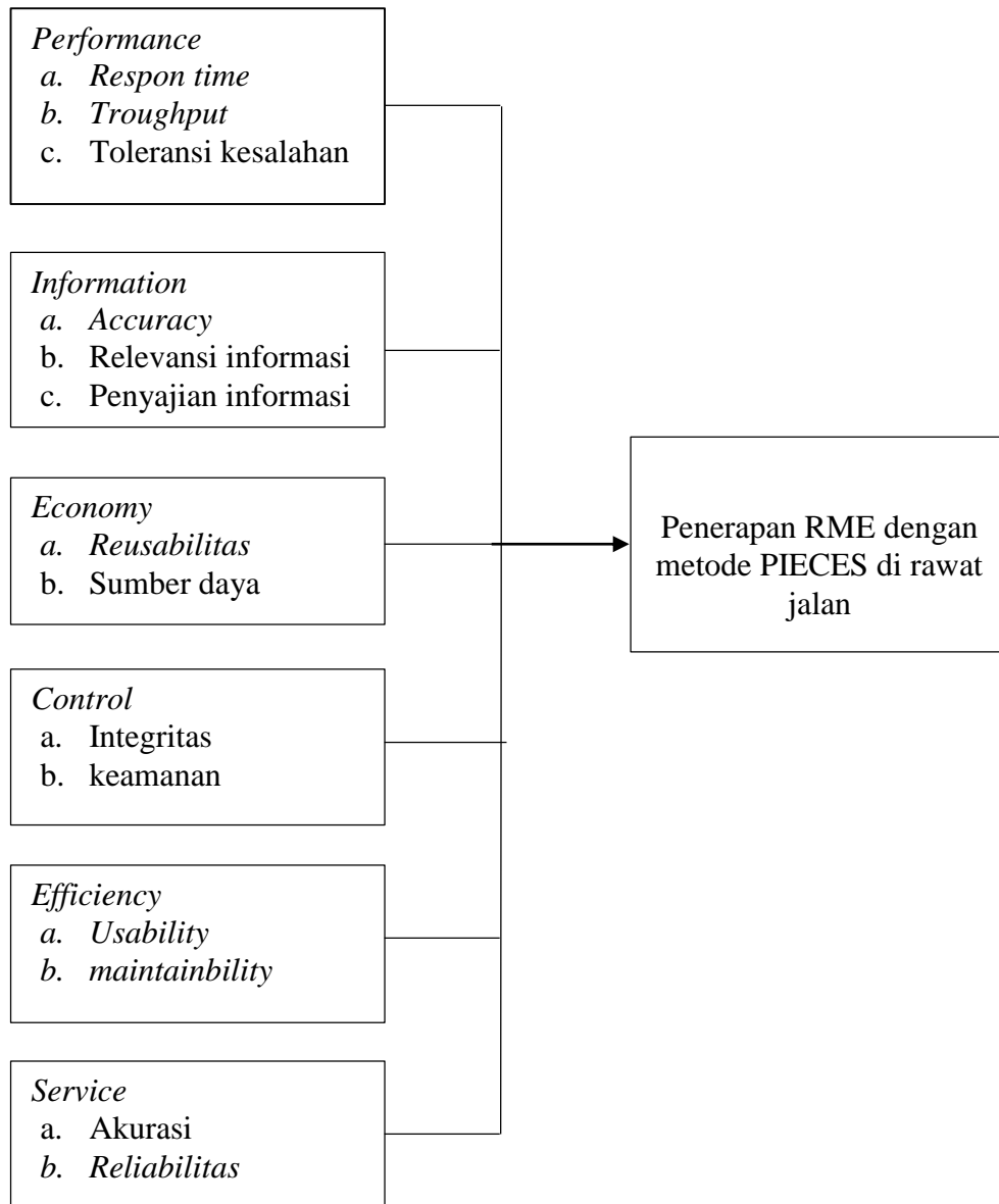
Gambar 3.1 Kerangka konseptual
