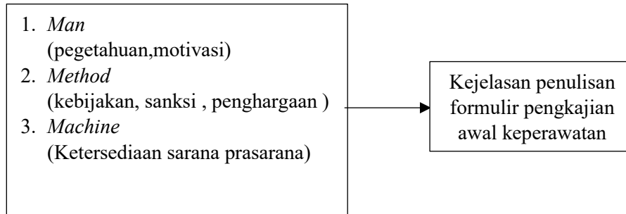
Gambar 3. 1 Kerangka Konseptual
