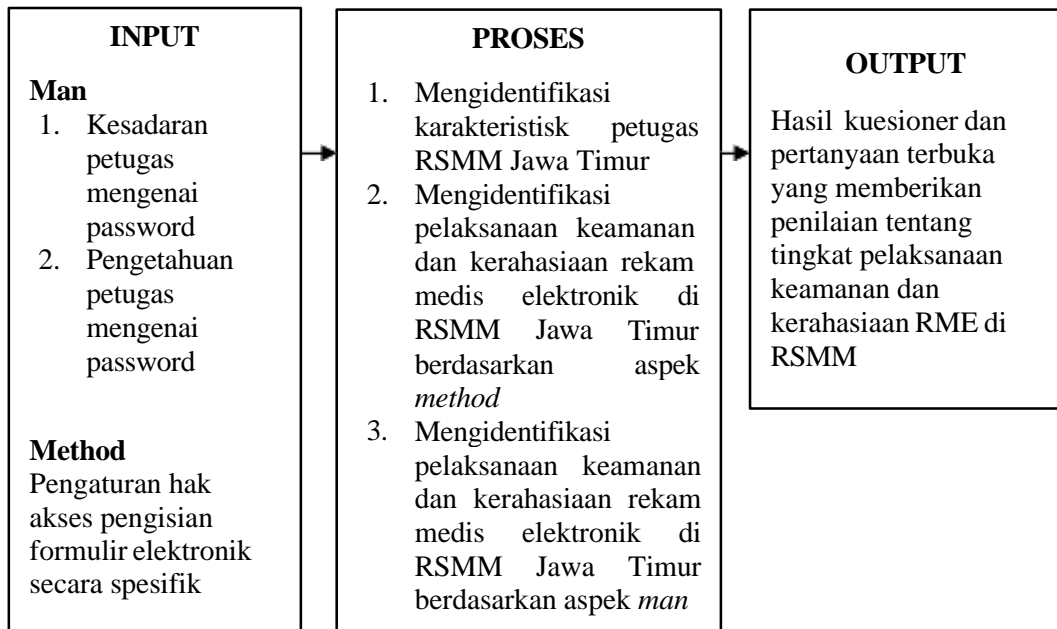
Gambar 3. 1 Kerangka Konseptual
